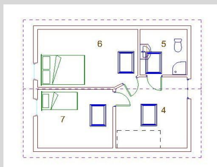
RZUT PODDASZA
